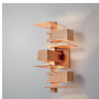
TALIESIN® 3 WALL SCONCE OAK 価格: 77,000円(税込) サイズ: H420×W192×D213mm 質量: 1.7kg 消費電力: 30W オーク塗装仕上
