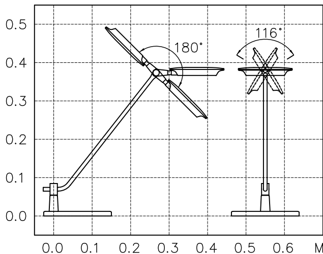
アーム・ヘッド可動範囲図
