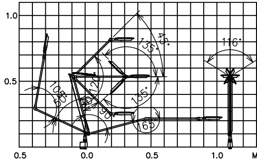
アーム・ヘッド可動範囲図
