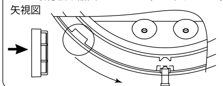
図 2 裏から見た場合は反時計回りに (○部の溝を下部のネジのところまで) 回転させ、取付板と器具カバーをはずしてください。
