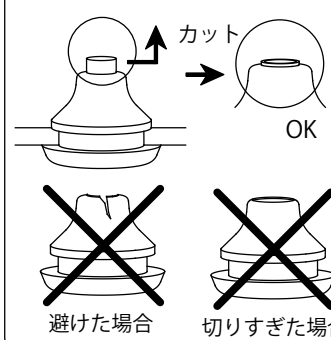
図 7 グロメット処理方法
