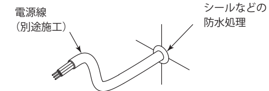
図2 電源線入り口の処理
