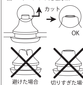
図4 グロメット処理方法
