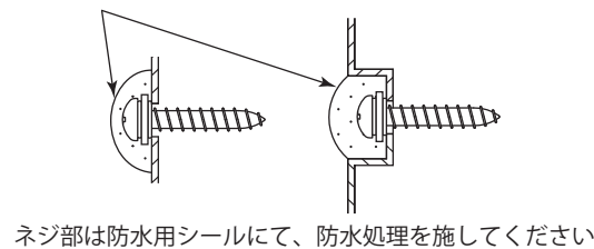
図3 防水用シールなどの防水処理
