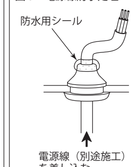
図5 電源線防水処理
