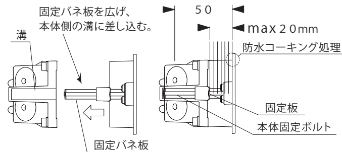
■ 埋込寸法図
