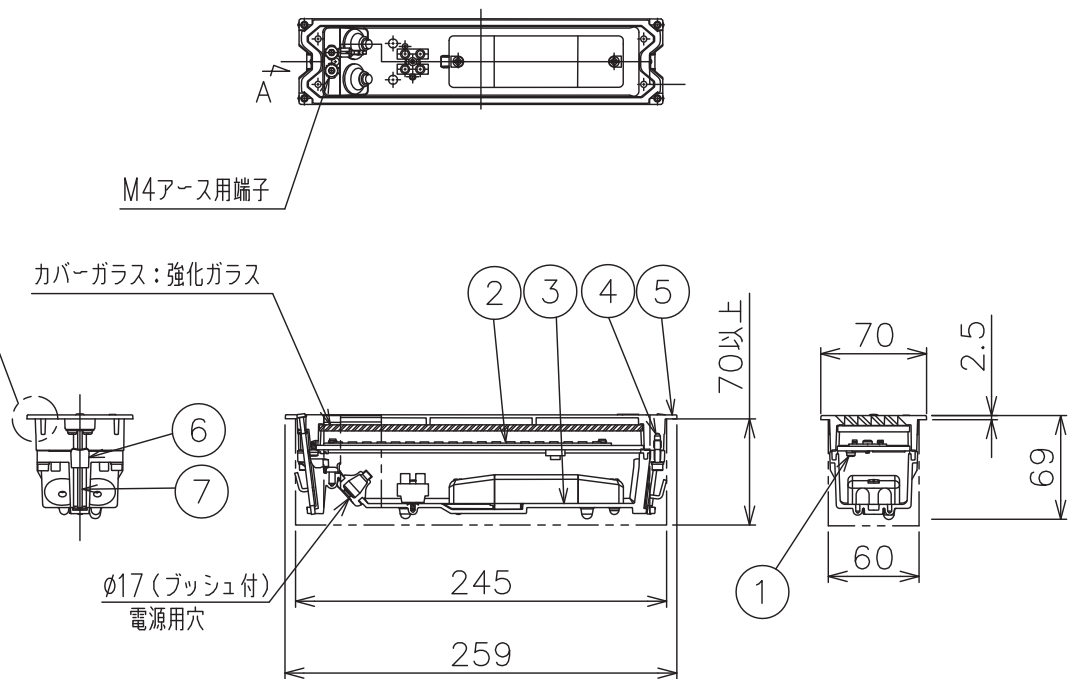
A矢視図
