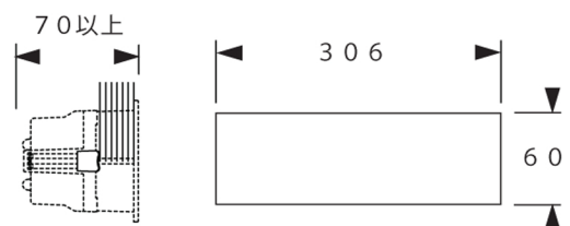
■ 埋込寸法図
