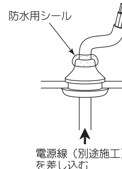
図6 電源線防水処理
