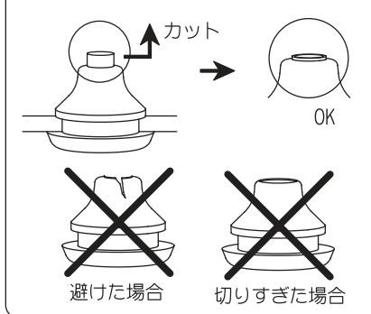
図5 グロメット処理方法
