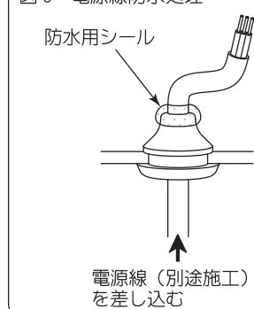
図6 電源線防水処理
