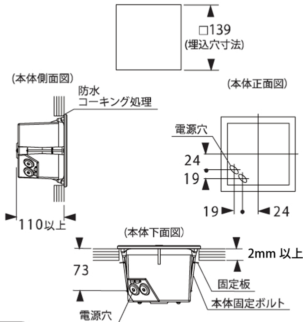
■ 埋込寸法図
