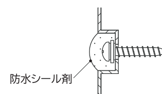
図5 取付ネジ部分の防水処理 ※防水用シール剤を使って防水処理をしてください。
