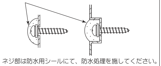
図4 防水用シールなどの防水処理
