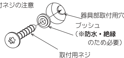
図2 取付ネジの注意
