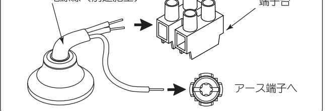
図7 電源線（別途施工）
