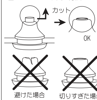
図5 グロメット処理方法
