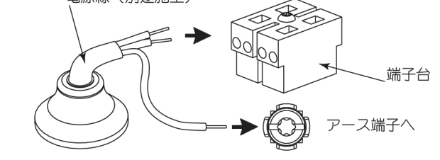
図 8 電源線（別途施工）
