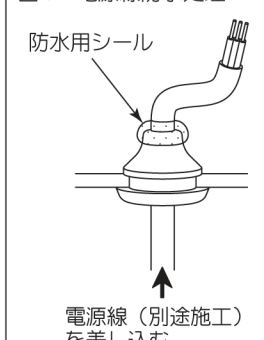
図 7 電源線防水処理
