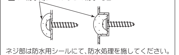
図5 防水用シールなどの防水処理
