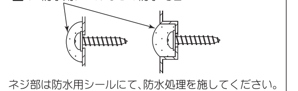
図5 防水用シールなどの防水処理
