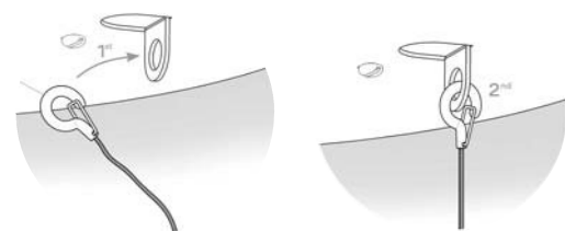
図1 仮吊ワイヤーの固定方法
