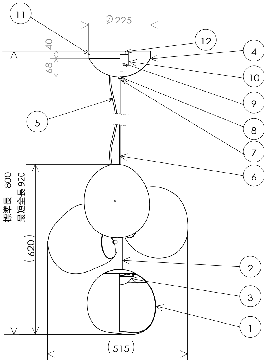
引掛け仕様(簡易取付け型)
