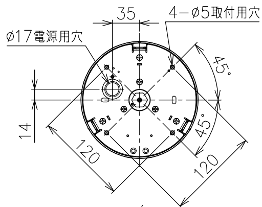
取付板詳細 S:1/5
