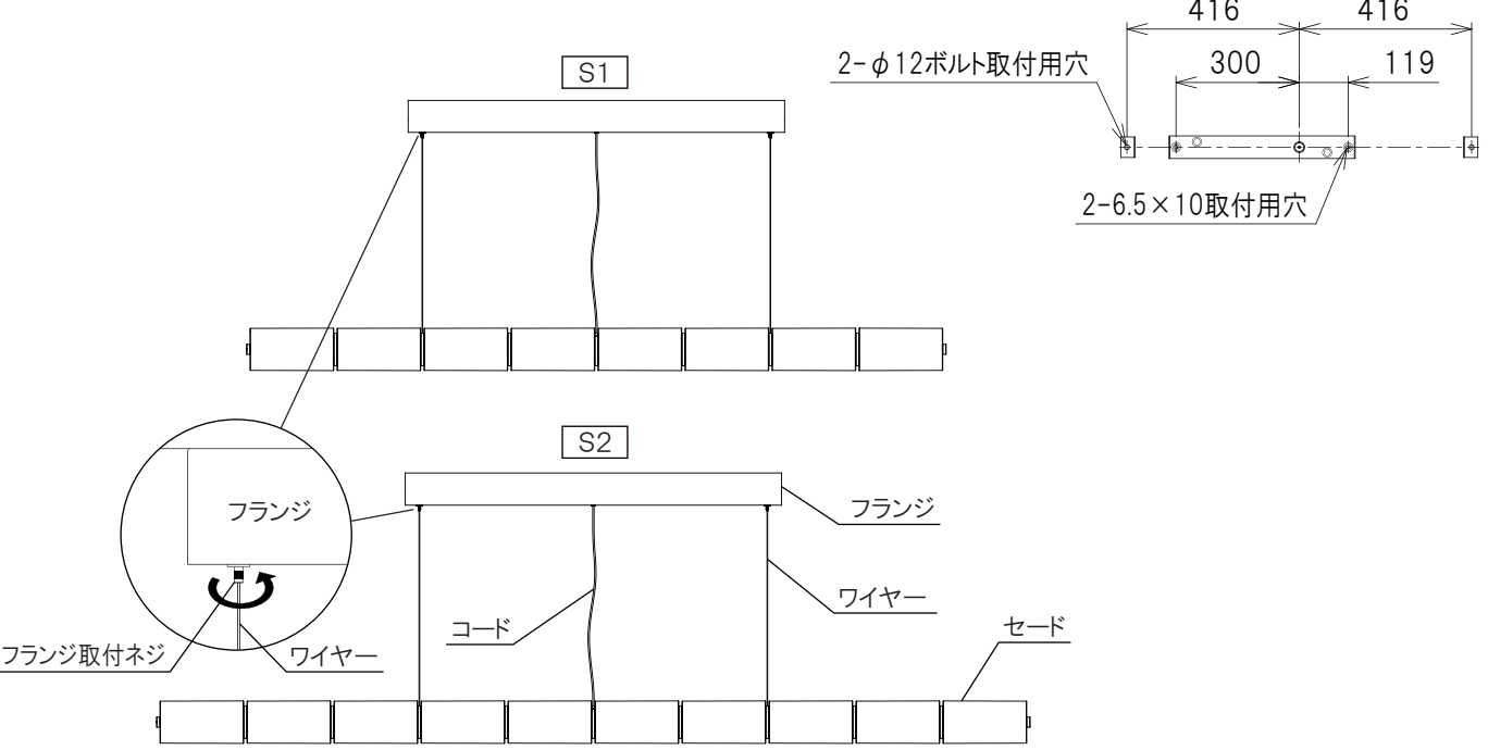
■取付ピッチ■
