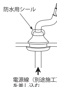
図 7 電源線防水処理
