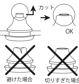
図 6 グロメット処理方法
