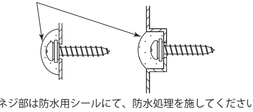
図 5 防水用シールなどの防水処理
