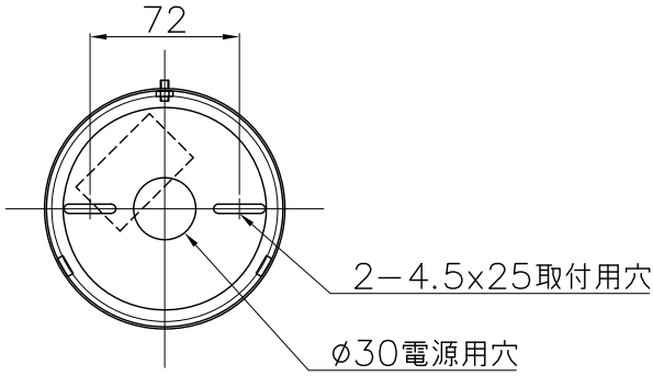
取付部詳細
