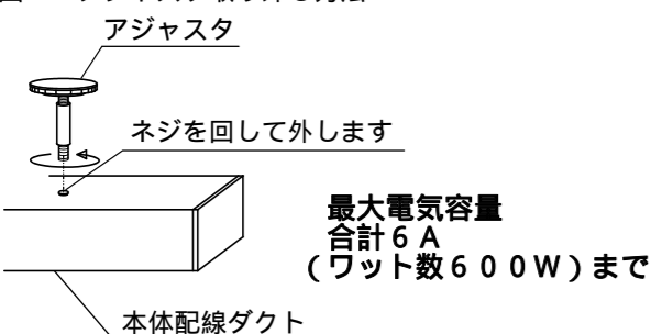
<図1> アジャスタ取り外し方法
