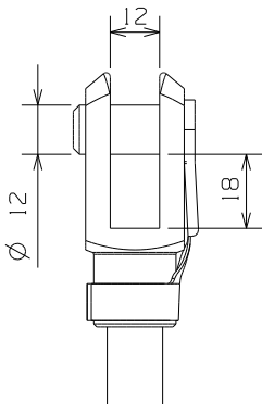
Detail beliere Echelle 1:2
