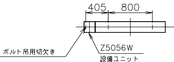
ボルト吊間隔寸法
