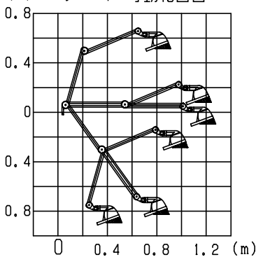
アームの可動範囲図
