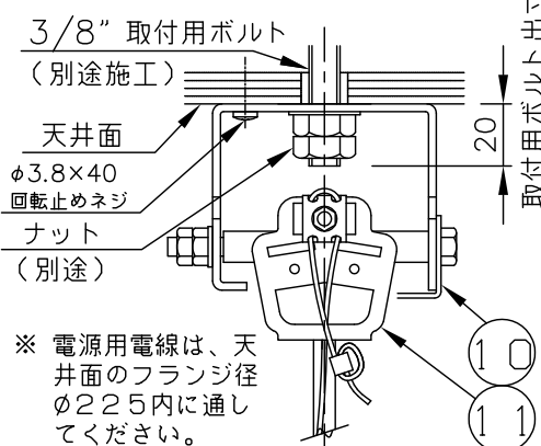
天井取付部詳細図
