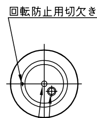
φ15取付ボルト用穴
