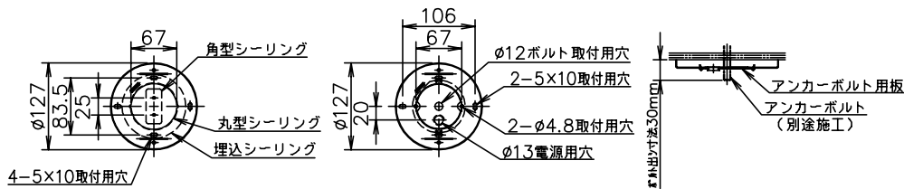
(A) 丸型・角型・埋込シーリングの場合 (付属のアンカーボルト取付用板は取り外してください。)
