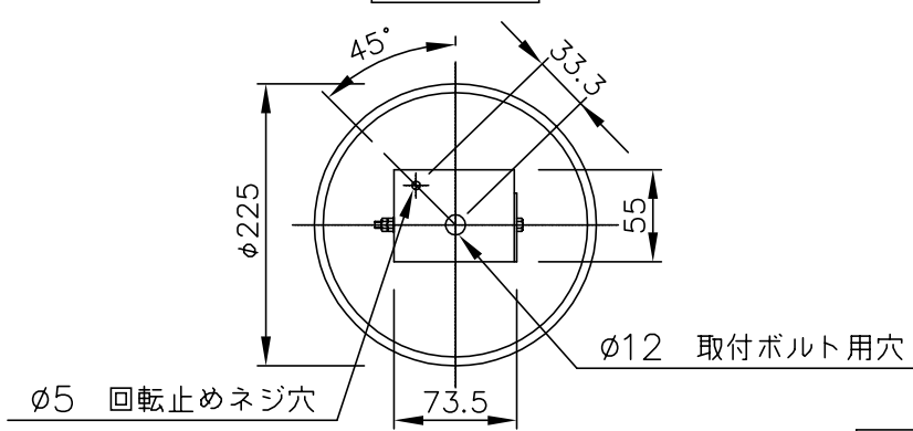
取付面図
