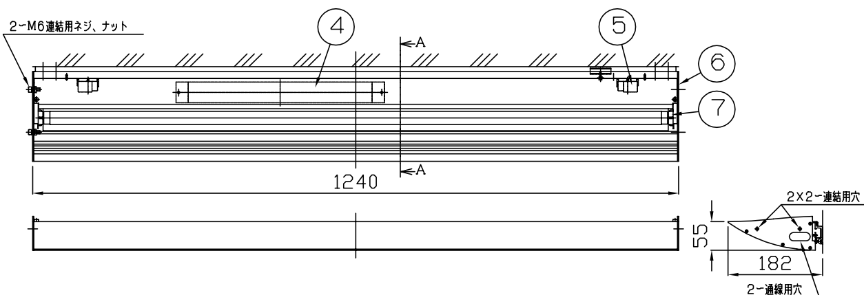
電源穴及び、取付穴寸法（壁面方向を見る）
