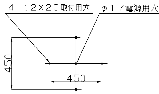
背面図
