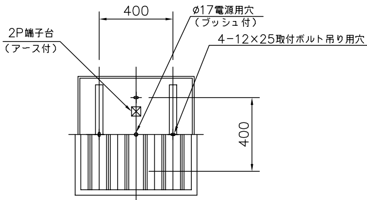
天井伏図
