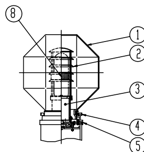
灯具部詳細
