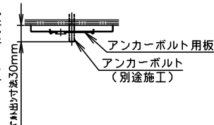
(B) ボルト又はボックスを使用する場合
