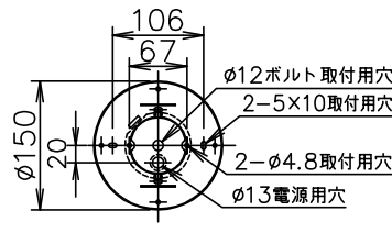
(B) ボルト又はボックスを使用する場合
