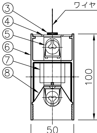
断面詳細図
