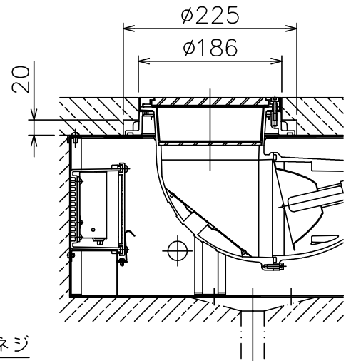
床材切込寸法参考図
