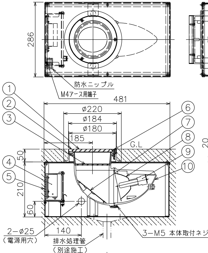
床材切込寸法参考図
