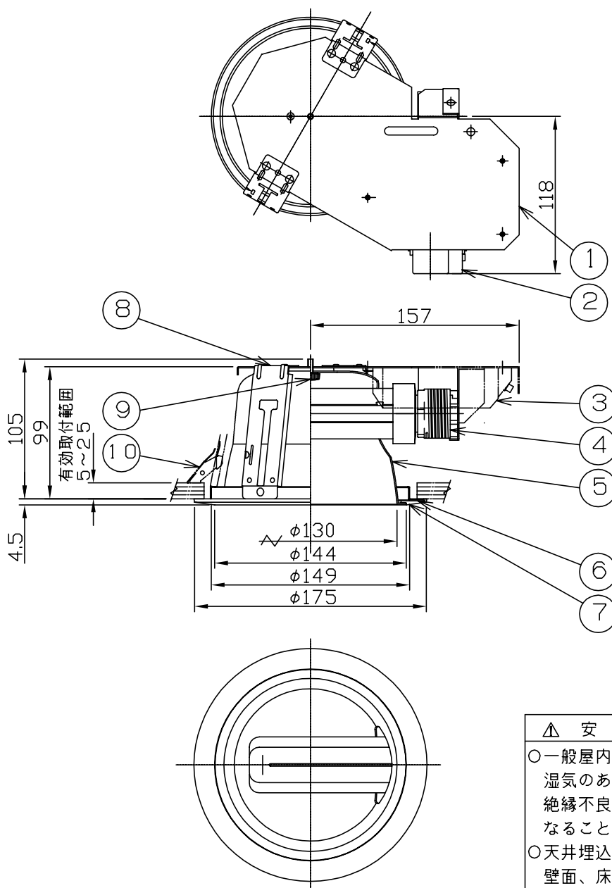
切込寸法
