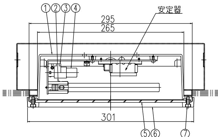
取付部分図
