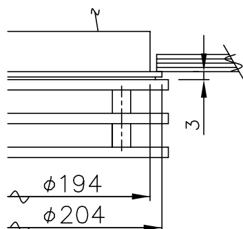
天井接触部詳細図
