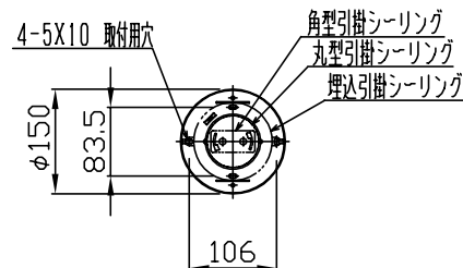
(A) 角型・丸型・埋込引掛シーリングの場合 (付属のアンカーボルト取付用板は取り外してください。)
