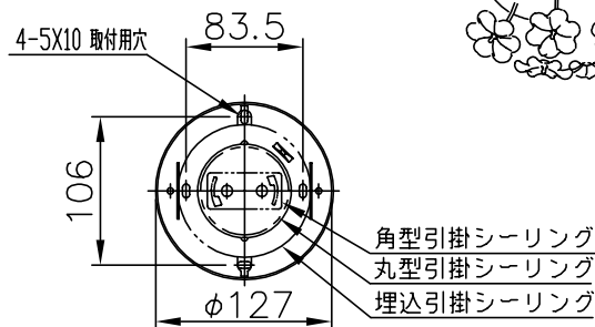
(A) 角型・丸型・埋込引掛シーリングの場合
