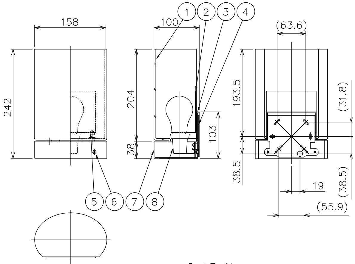
取付寸法詳細
