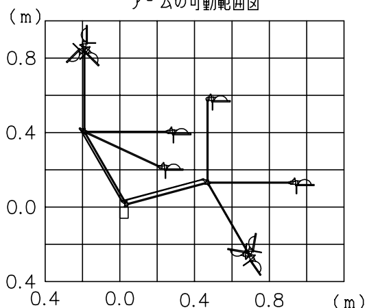
アームの可動範囲図
