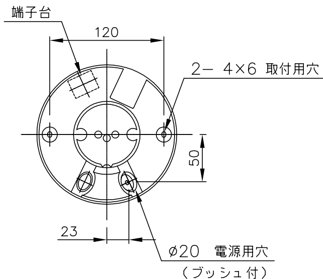
取付面図
