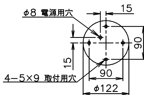
■取付ピッチ■
