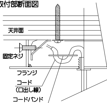
取付部断面図
