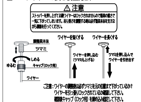
図1 ワイヤーの長さ調整方法
