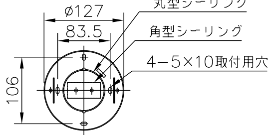
(A)丸型・角型・シーリングの場合
