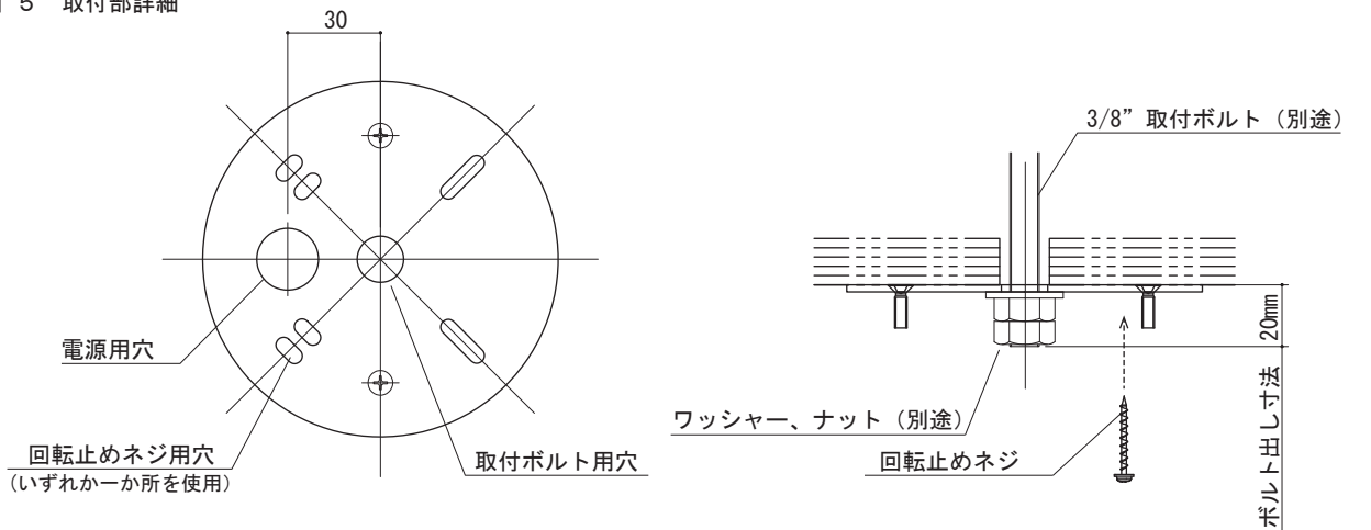
図 5 取付部詳細
